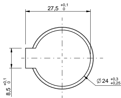
DETTAGLIO CAVA 1:1
