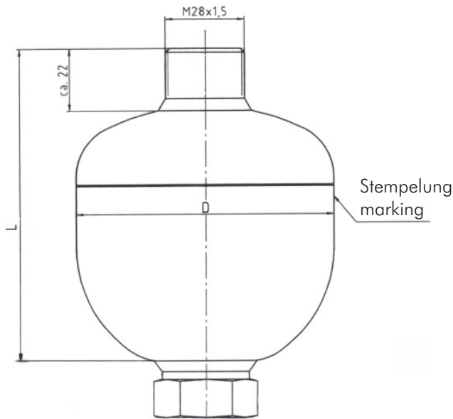
Ausführung 1 Design 1
